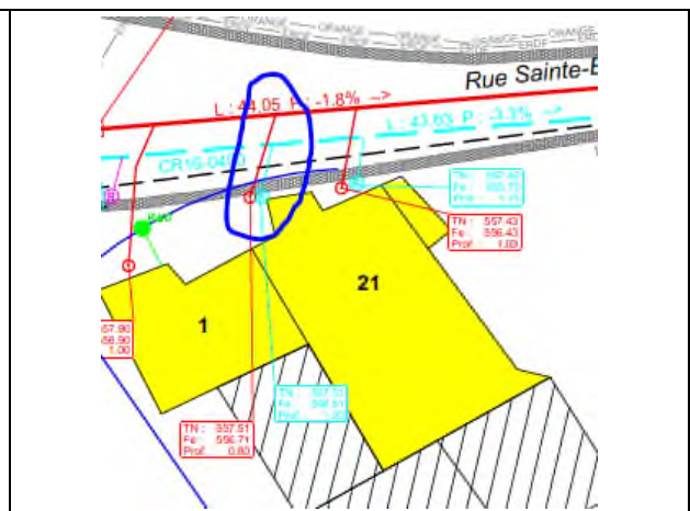
Boîtes de branchement à ne pas poser
