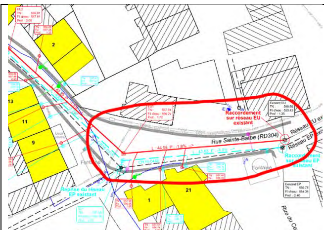
Réseau posé et croisement avec la conduite AEP
